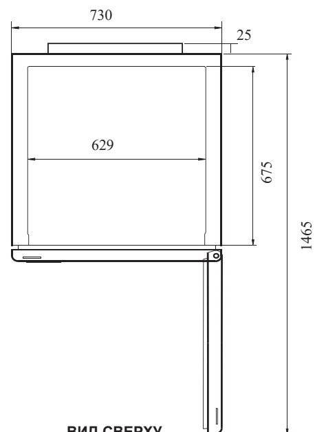
ВИД СВЕРХУ
